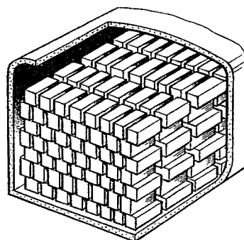
Шахматный способ укладки
