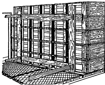
Вертикальный способ укладки
